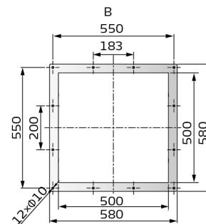
SGB-20XXX系列 底座安装尺寸
