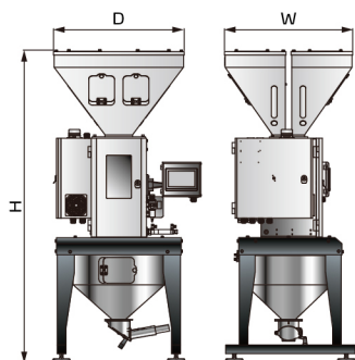
SGB-3XXX-GS系列(脚架安装型)
