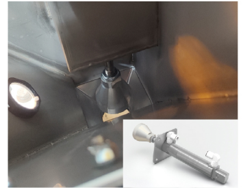
垂直计量阀
