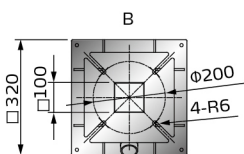
SGB-3XXX系列 底座安装尺寸
