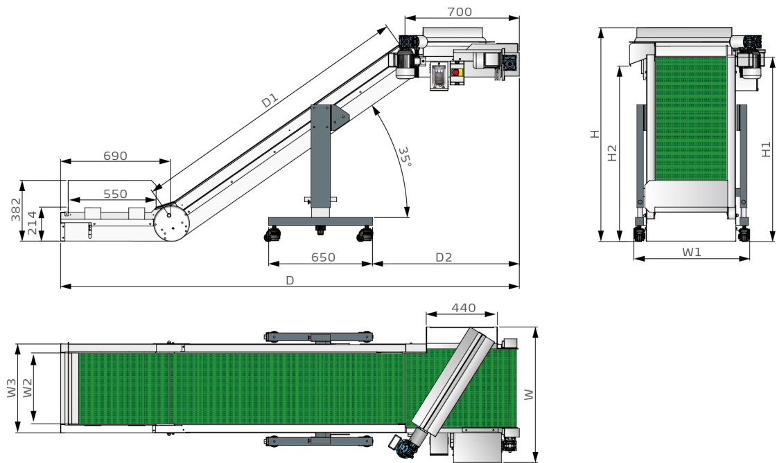
CBD 系列外形尺寸图
