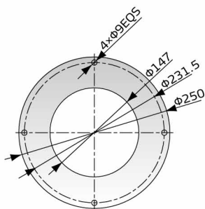
SHR-3U 安裝底座
