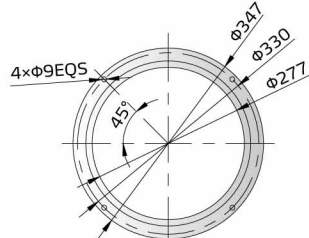
SLHR-36U-96U-S 安裝底座
