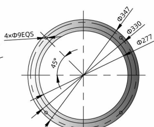
SHR-36U-S~SHR-96U-S 安装底座
