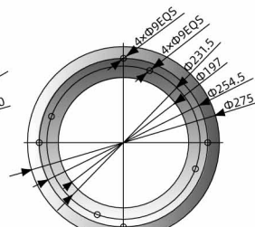
SHR-6U-S~SHR-24U-S 安装底座
