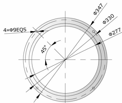
SHR-36U~120U 安裝底座
