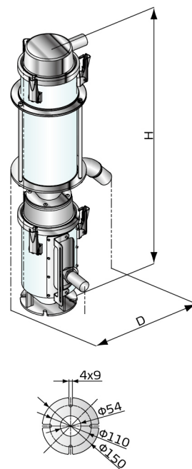
底座安装尺寸
