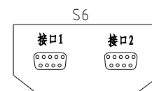
信易RS-485接口定义
