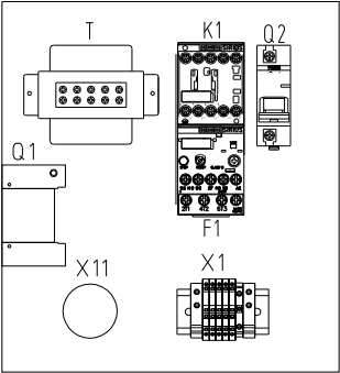
电控箱底板
