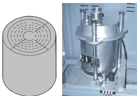
图 6-6: 蜂巢转轮图
