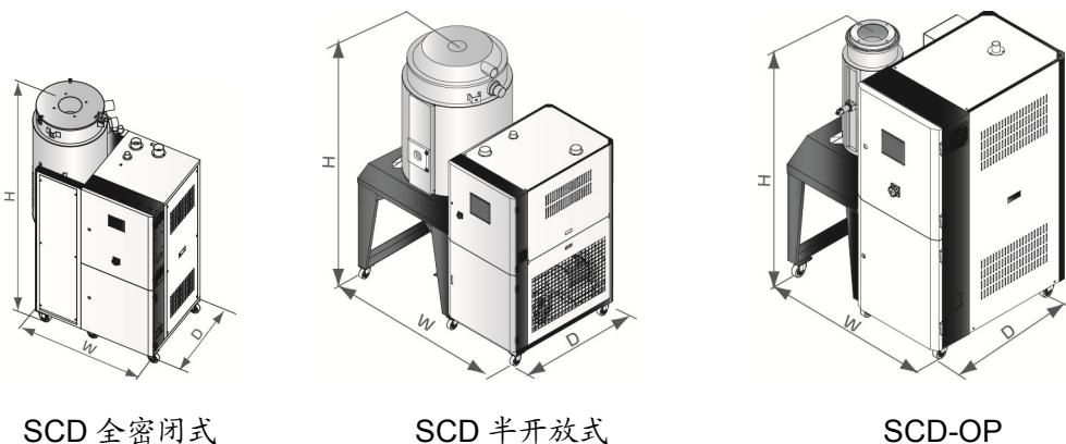
图 1-1: 外形尺寸图
