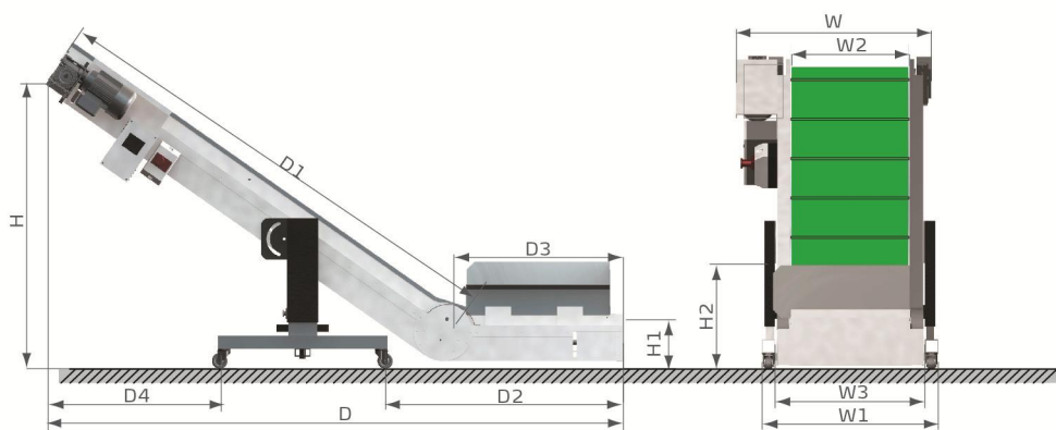
图 1-1: 外形尺寸图
